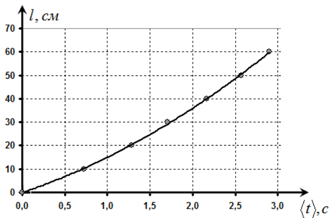
Рис.1 Скатывание цилиндра
