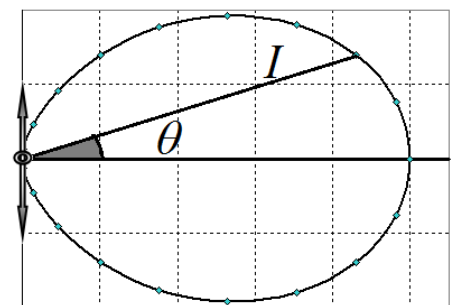
Индикатриса излучения дипольного излучателя
