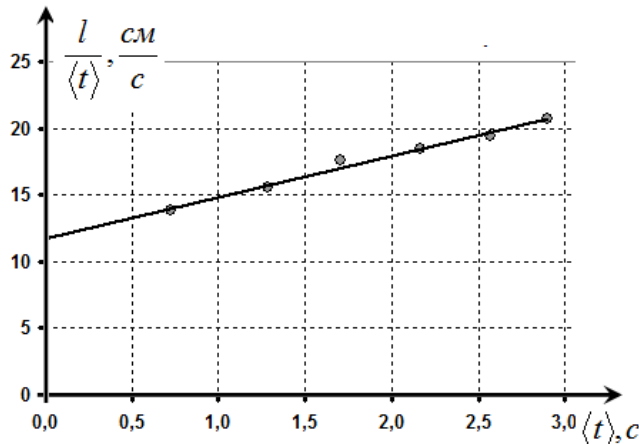
Рис.2 Скатывание цилиндра
