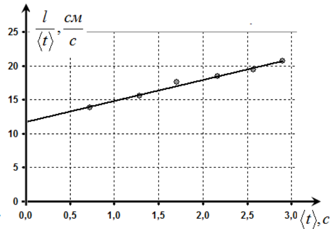
Рис.2 Скатывание цилиндра
