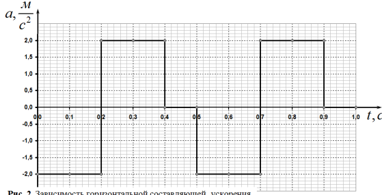
Рис. 2 Зависимость горизонтальной составляющей ускорения центра масс человека от времени.
