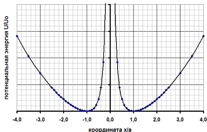
Зависимость потенциальной энергии от координаты
