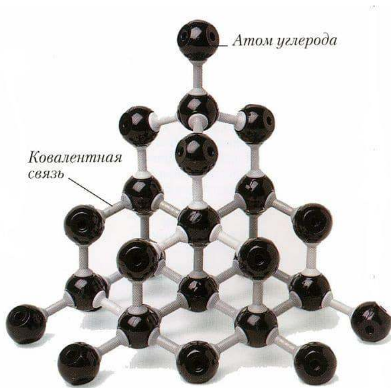
СТРУКТУРА АЛМАЗА
