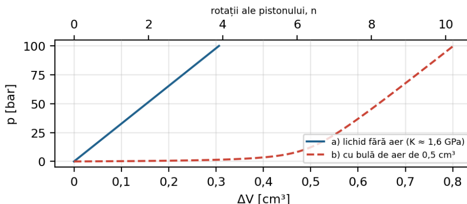
Fig. 2.2. Curba presiune – volum pentru lichidul fără aer și cu o bulă de aer de 0,5 \text{ cm}^3
