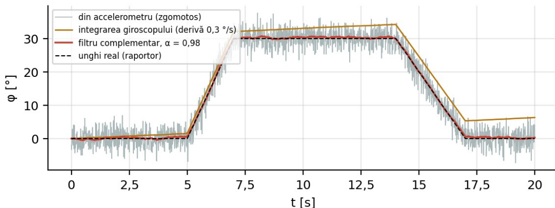
Fig. 8.1. Unghiul de rulu din accelerometru, din integrarea giroscopului și din filtrul complementar (simulare)
