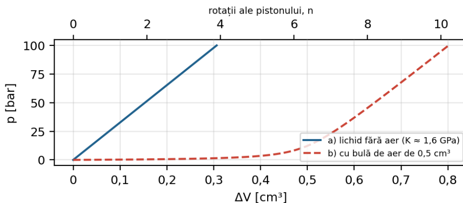
Fig. 2.2. Curba presiune – volum pentru lichidul fără aer și cu o bulă de aer de 0,5 \text{ cm}^3
