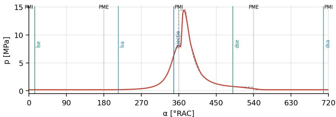
Fig. 11.2. Diagrama indicată desfășurată p-α, cu fazele distribuției (MAC)
