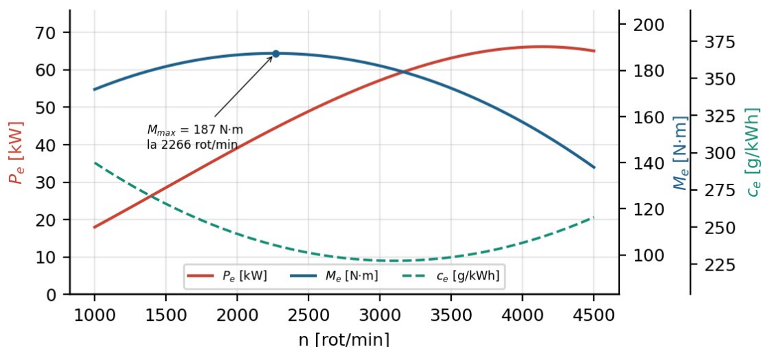
Fig. 11.4. Caracteristica exterioară de turație (MAC)
