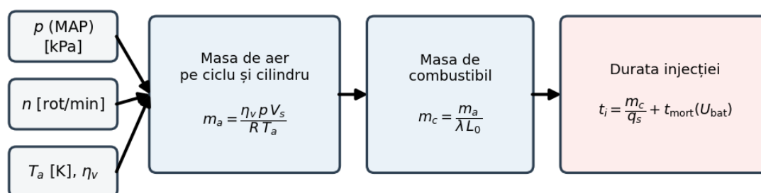
Fig. 2.1. Structura modelului de calcul al duratei de injecție
