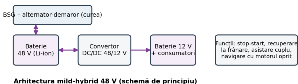
Fig. 7.4. Arhitectura mild-hybrid 48 V (schemă de principiu)
