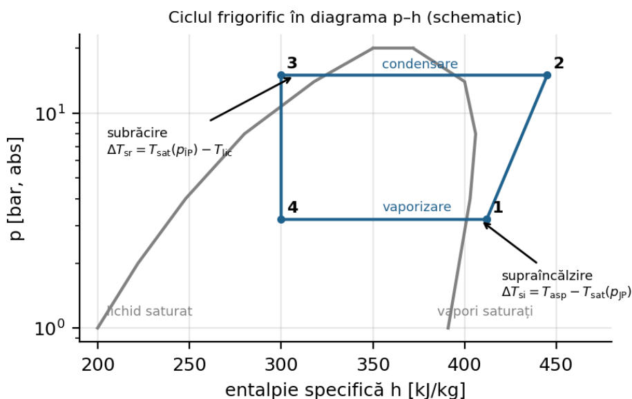
Fig. 8.2. Ciclul frigorific în diagrama presiune-entalpie (schematic)
