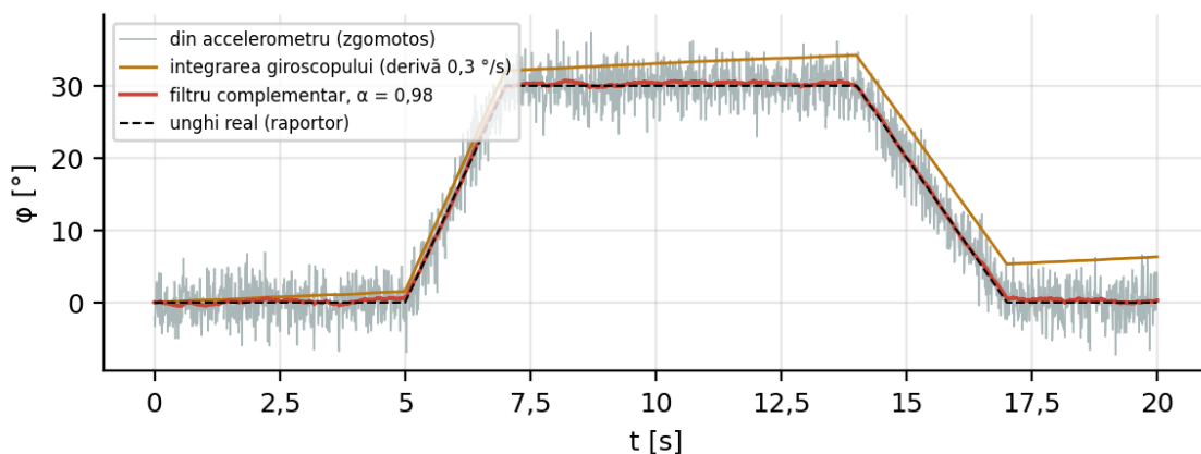
Fig. 8.1. Unghiul de rulu din accelerometru, din integrarea giroscopului și din filtrul complementar (simulare)
