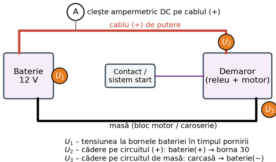
Fig. 7.1. Circuitul de pornire și punctele de măsură
