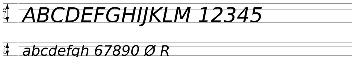
Fig. 6. Linii ajutătoare și exemplu de scriere înclinată ( h = 10 și h = 7 mm)
