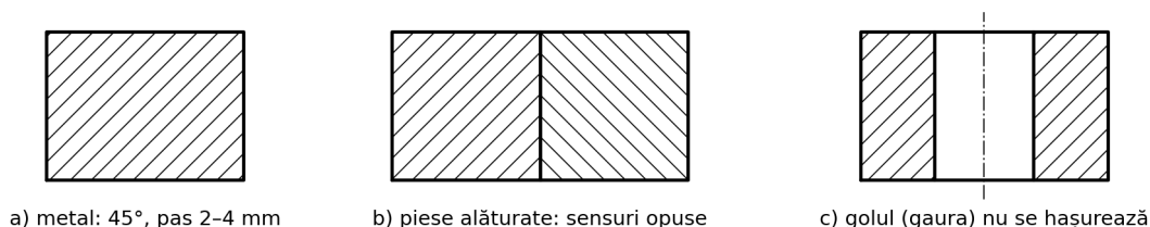
Fig. 12. Reguli de hașurare
