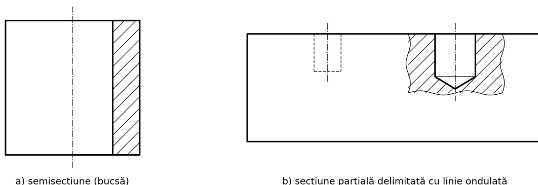
Fig. 14. Semiseccțiune și secțiune parțială
