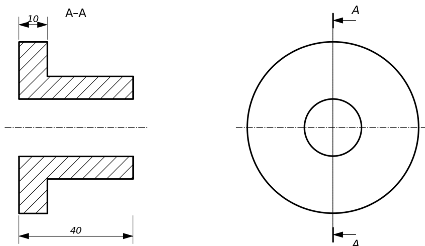
Fig. 13. Bucșă cu guler: secțiunea A-A și vederea laterală cu traseul de secționare
