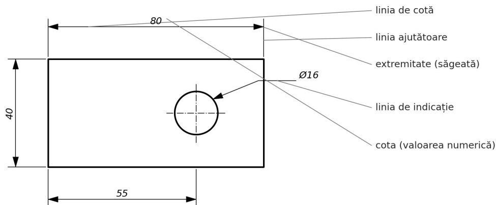
Fig. 17. Elementele cotării
