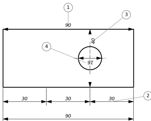
Fig. 20. Exercițiu: găsește greșelile de cotare marcate 1...4
