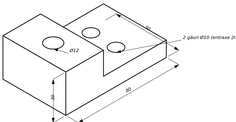
Fig. 21. Placă de ghidare – dimensiuni de gabarit, găuri și treaptă
