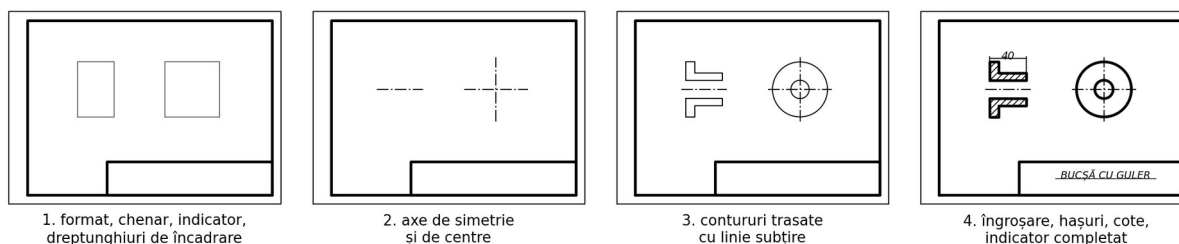
Fig. 27. Etapele executării schiței (bucșă cu guler, secțiune + vedere laterală)
