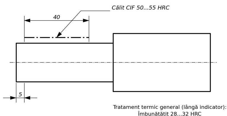
Fig. 35. Zonă tratată termic marcată cu linie punct groasă; tratament general lângă indicator
