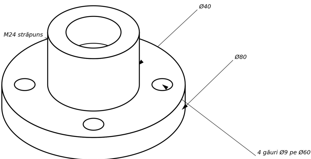
Fig. 38. Flanșă cu butuc filetat: flanșă \text{Ø}80 \times 12 cu 4 găuri \text{Ø}9 pe \text{Ø}60 ; butuc \text{Ø}40 \times 28 ; gaură filetată M24 străpunsă
