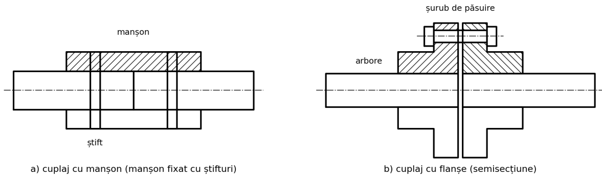
Fig. 13. Cuplaje fixe
