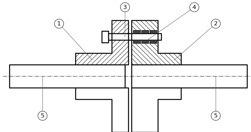
1 - semicuplaj cu bolțuri; 2 - semicuplaj cu alezaje; 3 - bolț; 4 - inele (bucșe) de cauciuc; 5 - arbori Inelele elastice preiau șocurile și mici abateri de coaxialitate.
