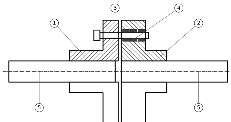
Fig. 13. Cuplaje fixe
