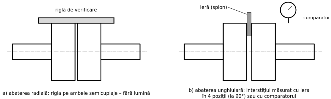
Fig. 15. Verificarea alinierii arborilor la cuplaje
