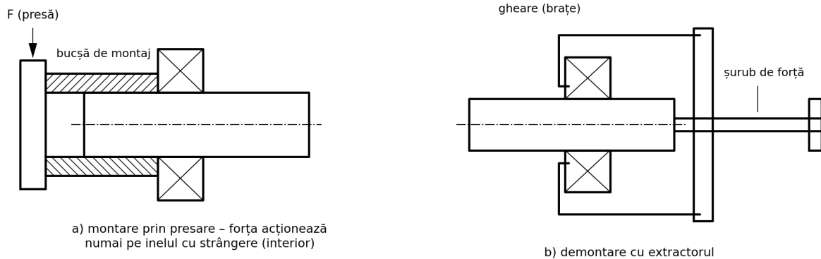
Fig. 20. Montarea și demontarea rulmenților
