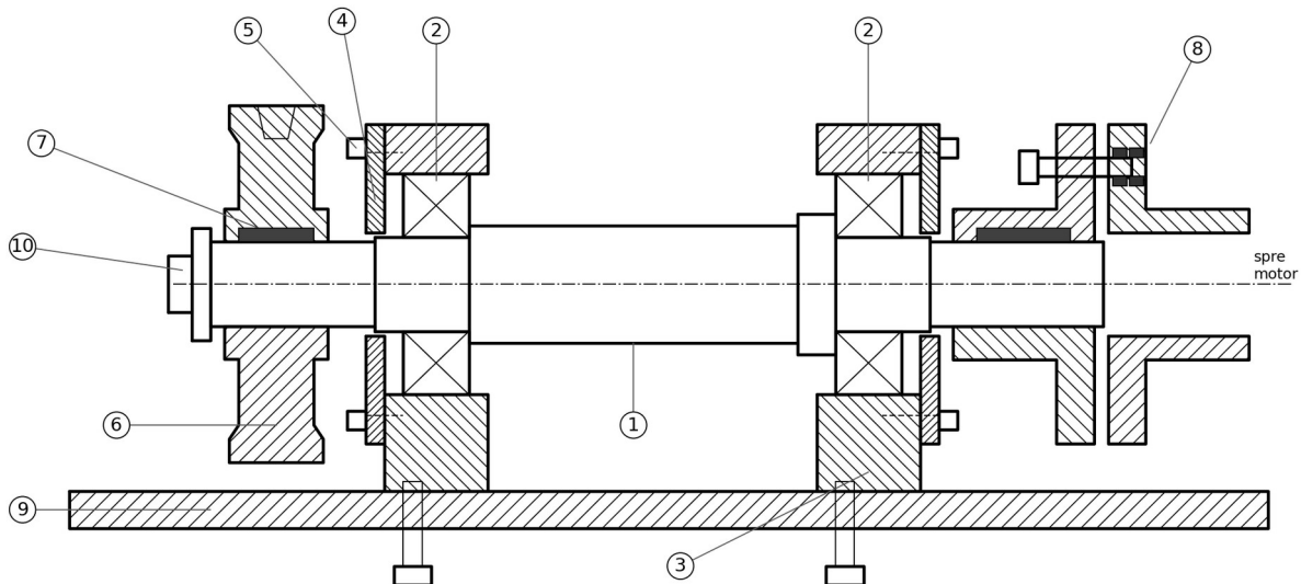
Fig. 24. Standul de transmisie – subansamblul probei practice E7
