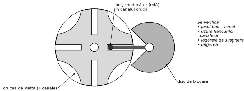
Fig. 15. Mecanismul cu cruce de Malta cu 4 canale
