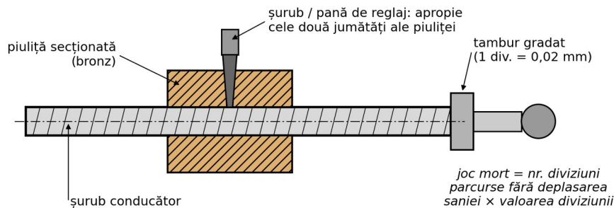
Fig. 16. Mecanismul șurub-piuliță cu piuliță secționată reglabilă
