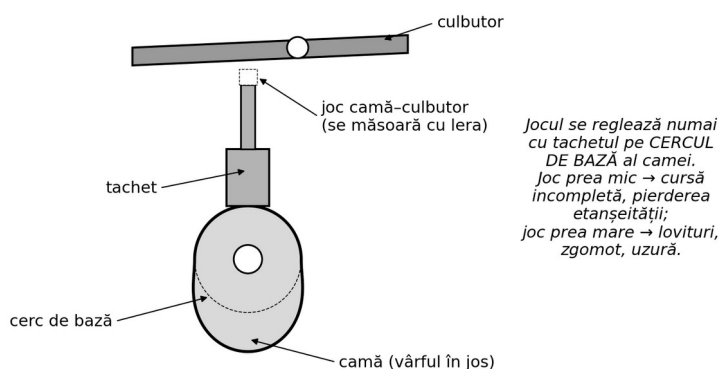
Fig. 14. Mecanismul cu camă, tachtet și culbutor; jocul se reglează pe cercul de bază
