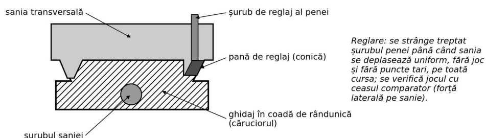
Fig. 19. Sania transversală cu ghidaj în coadă de rândunică și pană de reglaj conică
