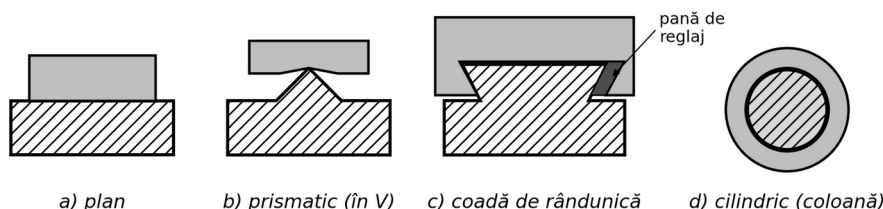
Fig. 18. Formele ghidajelor de alunecare
