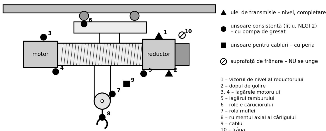
Fig. 15. Schema de ungere a electropalanului (model)
