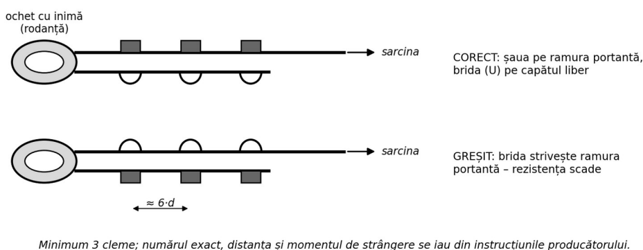
Fig. 18. Montarea corectă și greșită a clemelor pe cablu
