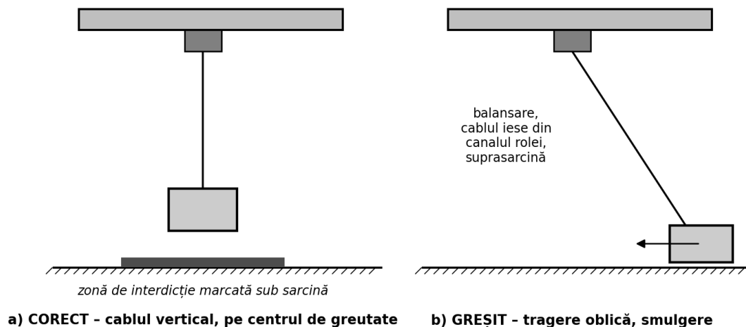
Fig. 21. Ridicarea corectă (verticală) și cea greșită (oblică)
