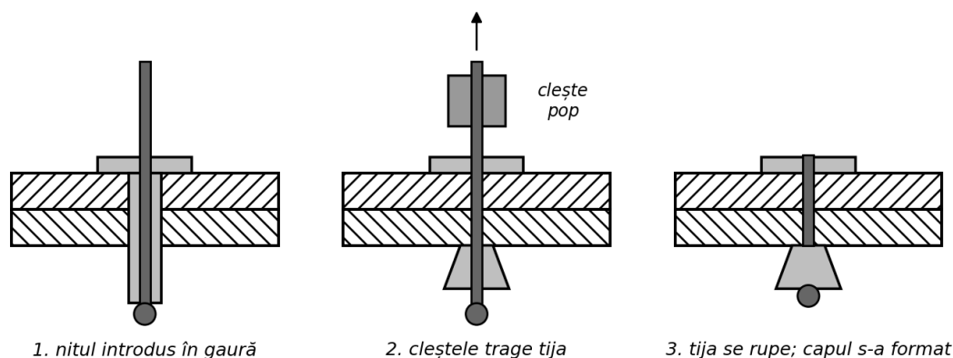
Fig. 8. Nituirea cu nit orb (pop)
