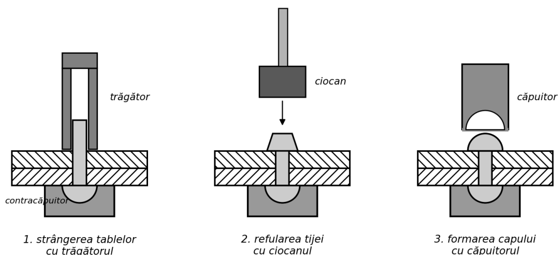
Fig. 7. Fazele nituirii manuale cu nit cu cap semirotund
