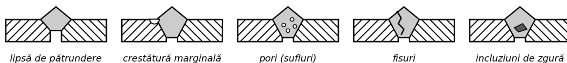
Fig. 12. Defecte ale îmbinărilor sudate
