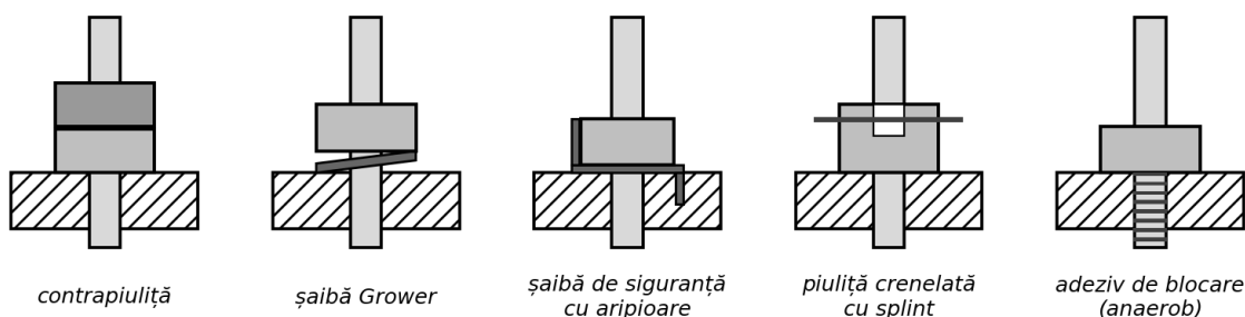
Fig. 18. Asigurarea piulițelor împotriva autodesfacerii
