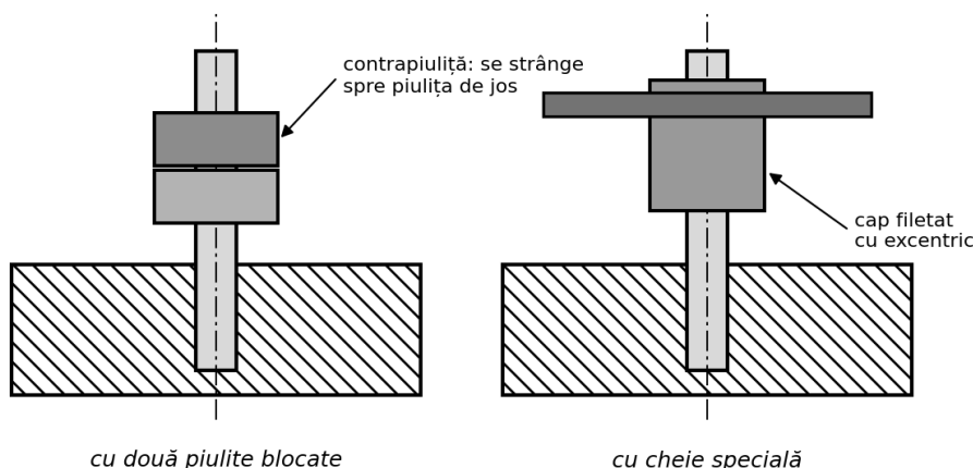
Fig. 19. Montarea prezoanelor
