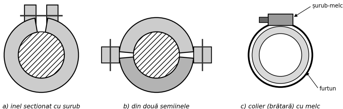
Fig. 25. Brățări: a – inel secționat cu șurub; b – din două semiinele; c – colier cu melc
