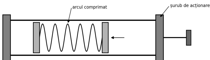
Dispozitiv (presă) cu șurub pentru precomprimarea arcurilor
