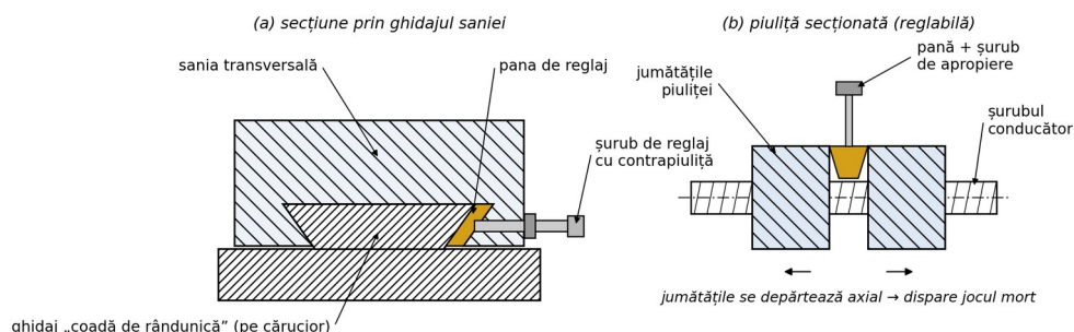
Fig. 17. Pana de reglaj a saniei și piulița secționată a șurubului transversal
