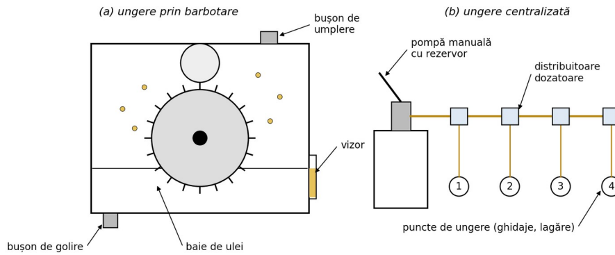
Fig. 28. Ungerea prin barbotare și ungerea centralizată
