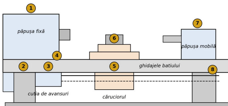
Fig. 27. Schema de ungere simplificată a unui strung (numerotarea punctelor – exemplu)
