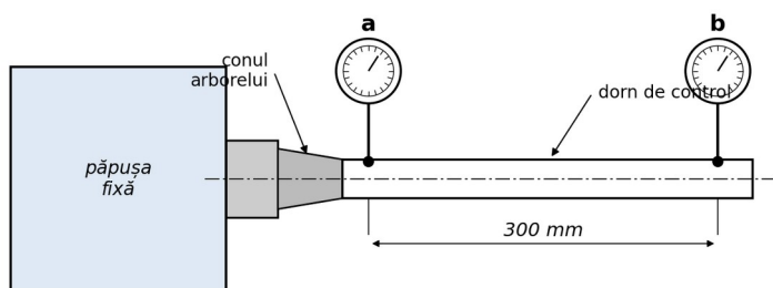
Fig. 30. Verificarea bătaii radiale a arborelui principal cu dorn de control
