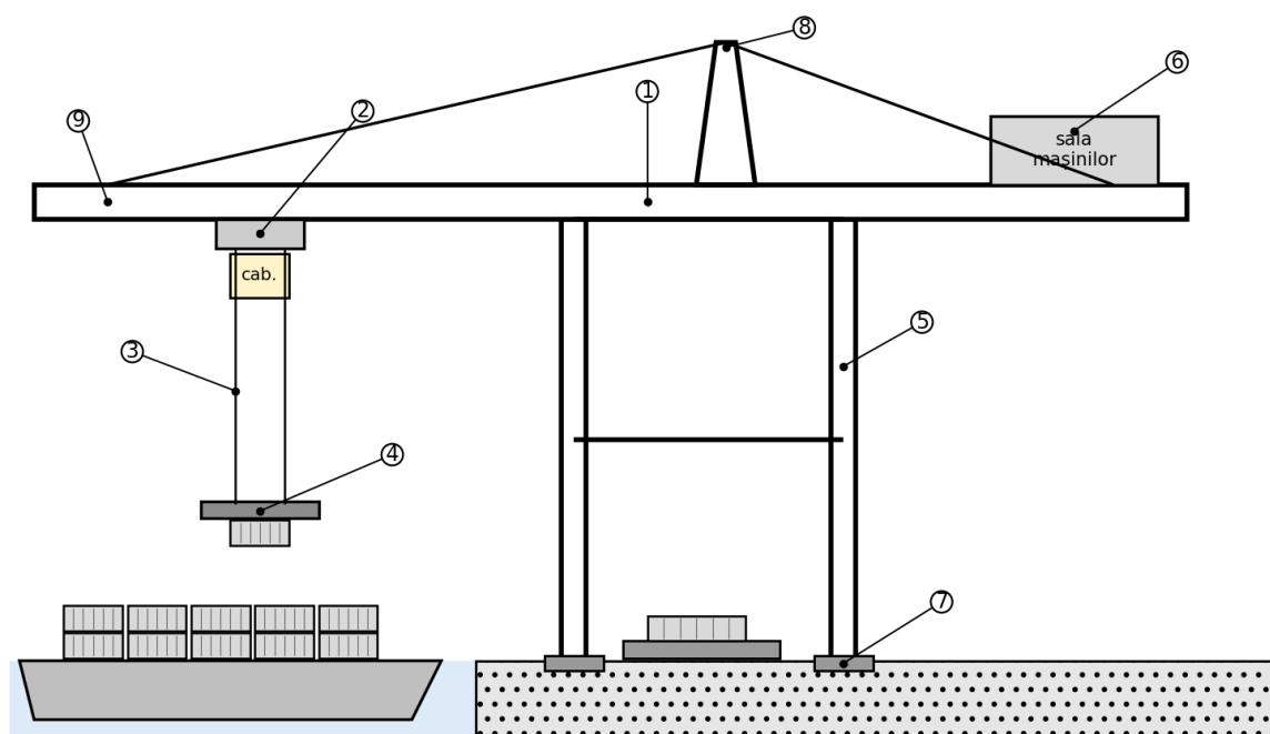
1 grindă principală · 2 cărucior cu cabina macaragiului · 3 cabluri de ridicare · 4 spreader · 5 picior de portal 6 sala mașinilor (ridicare, deplasare cărucior) · 7 boghiuri de translație pe șine · 8 turn (A-frame) · 9 braț rabatabil (boom)
