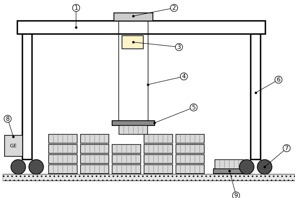
1 grindă transversală · 2 cărucior · 3 cabina macaragiului · 4 cabluri de ridicare · 5 spreader · 6 picior de portal 7 roți cu pneuri (boghiuri, direcție) · 8 grup electrogen / alimentare · 9 tractor de terminal pe banda de circulație
