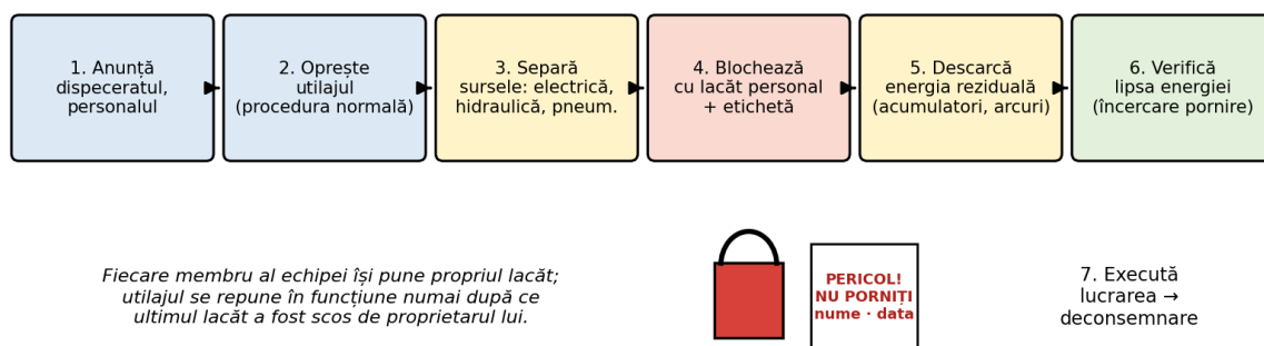
Fig. 9. Consemnarea utilajului înainte de intervenție (LOTO) – succesiunea generică
