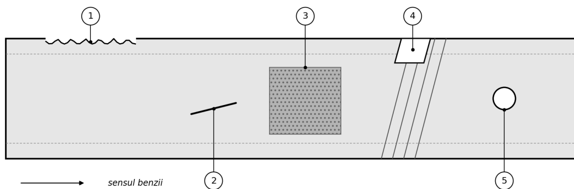
Fig. 4. Defecte ale benzii (vedere de sus): 1 margine uzată / ruptă; 2 fisură transversală; 3 uzura stratului de acoperire; 4 îmbinare cu desprindere; 5 lovitură / perforare de la un corp străin
