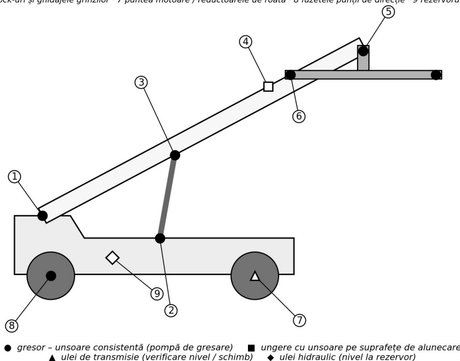
Fig. 10. Schema de ungere a unui reach-stacker – puncte-tip (schemă didactică; punctele reale se iau din cartea tehnică)
