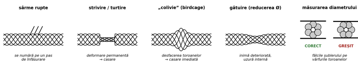
Fig. 15. Defecte ale cablurilor de oțel și măsurarea corectă a diametrului
